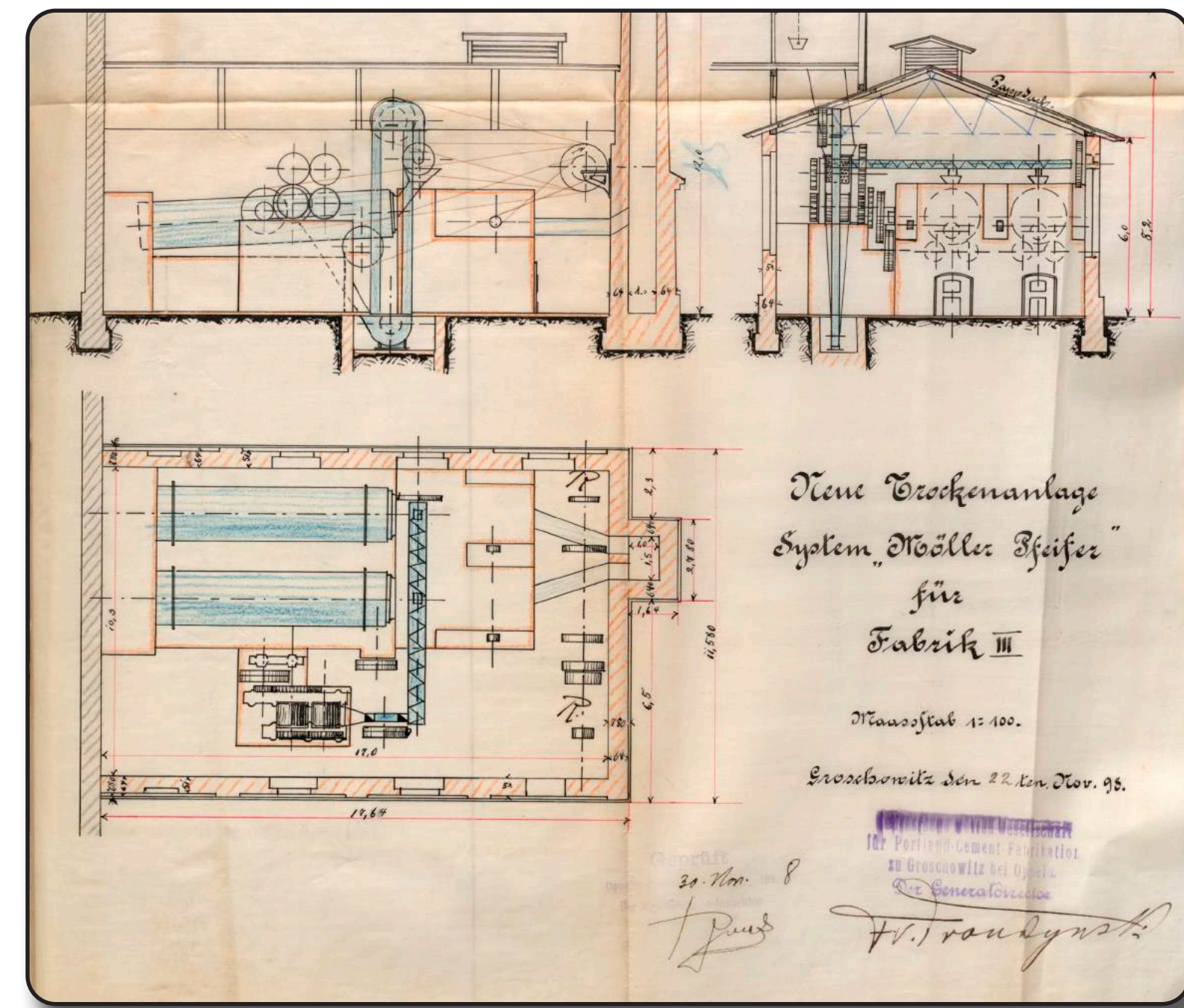
Szkice projektowe urządzeń suszarni.
