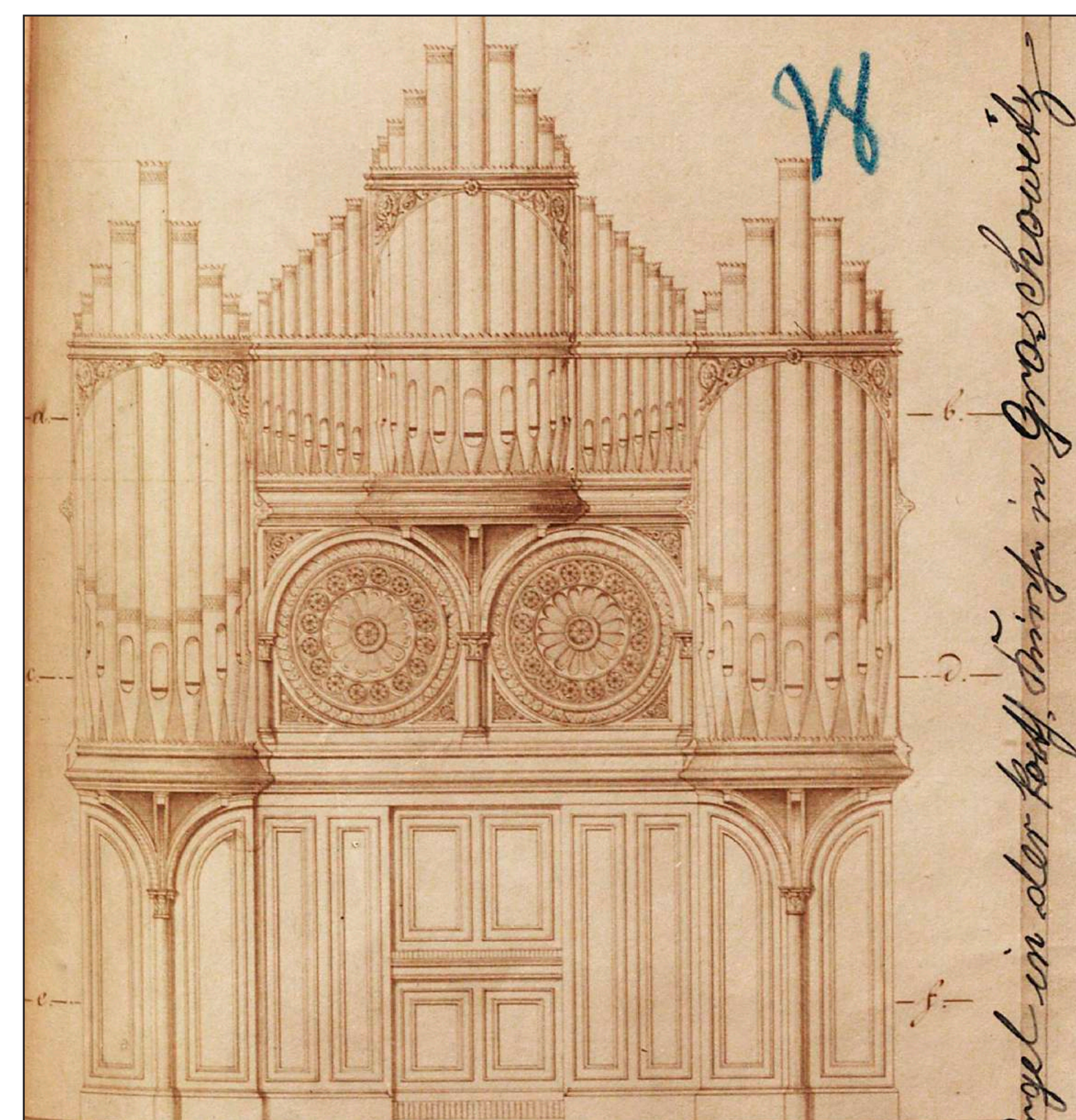
Szkic inwentaryzacyjny kościelnych organów sporządzony na potrzeby renowacji w 1913 r.
